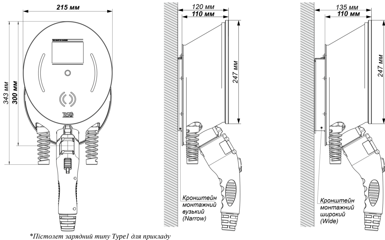
Рис.2 - Габарити та загальний розмір зарядного пристрою для електроавтомобіля
